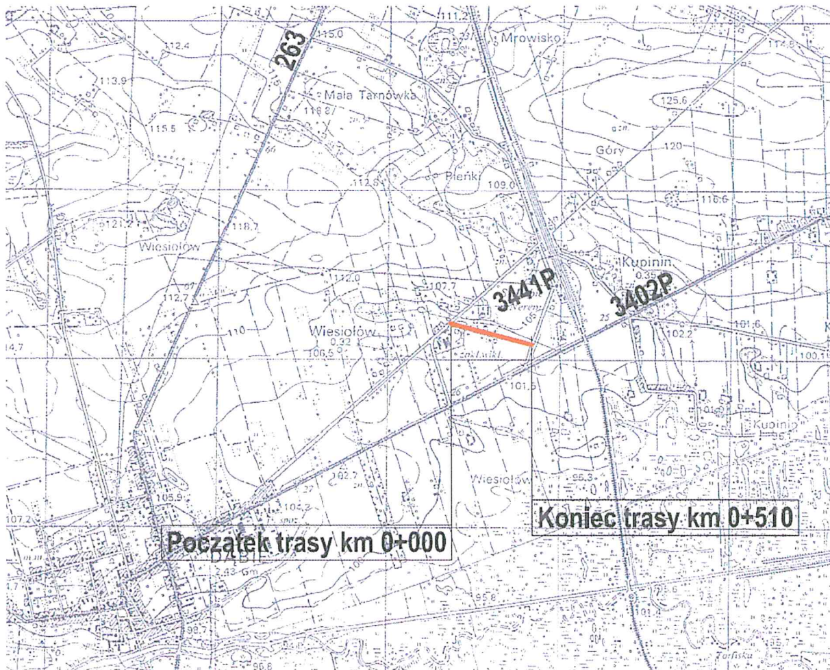
Przebieg drogi w miejscowości Wiesiołów
